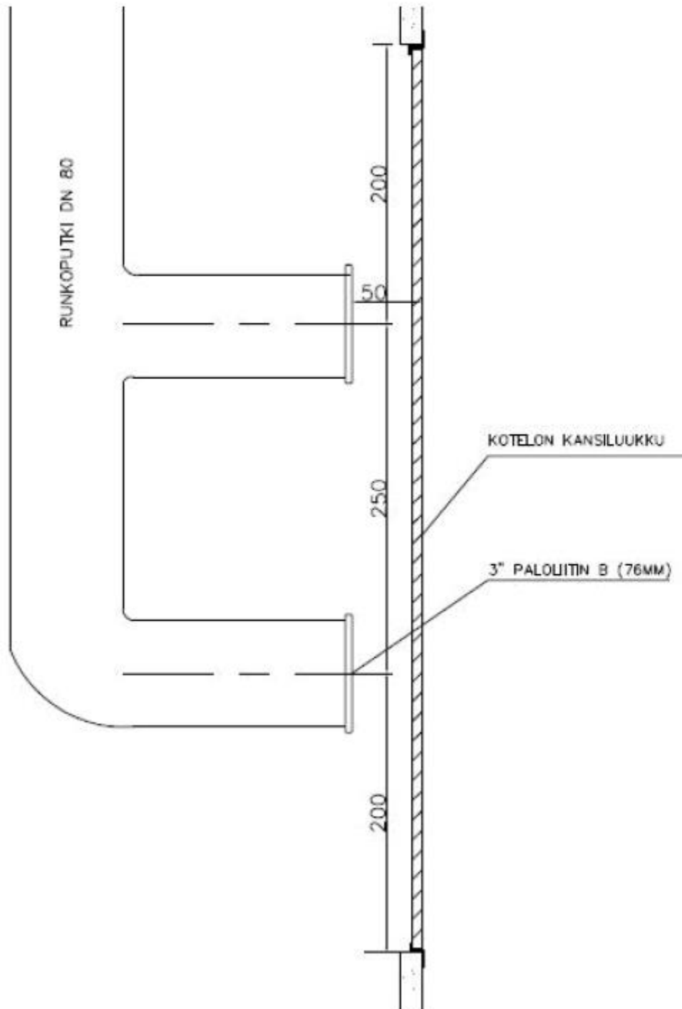
Kuva 4. Vedensyöttöliittimet kuvattuna sivusta, 2 x 3":n paloliitin B. Varustettava ohjeen tekstiosan mukaisilla yksisuunta- ja tyhjennysventtiileillä (ei näy kuvassa).
